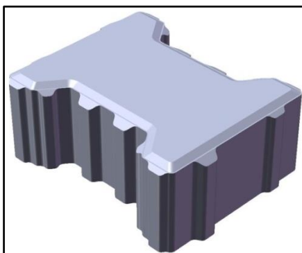
Aquaflow H-profiel steen met waterpassage 200*165*100mm (35,7 st/m 2 )
