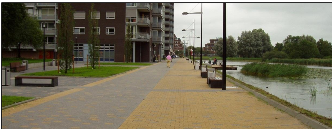
> 100 m 3 waterberging onder de parkpromenade met vertraagde afvoer naar oppervlakte water.
