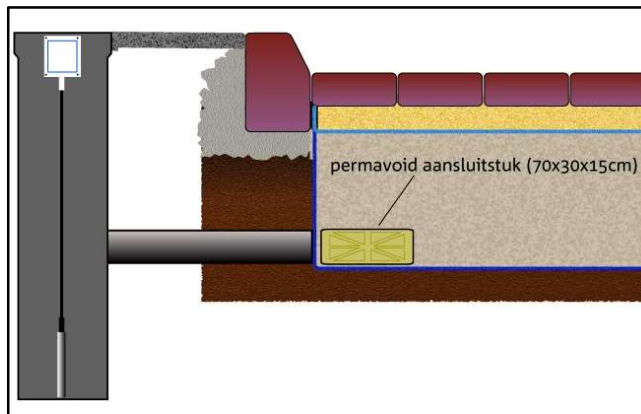
Flowfacts wordt in een putje geplaatst en verbonden met de waterbergende weg.
